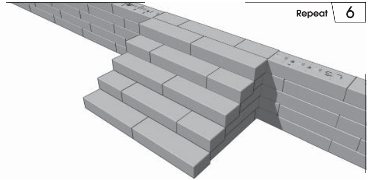
Geogrid Layer 4
